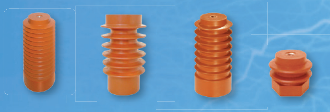
Traversée-isolateurs de 7,2 kV à 42 kV
